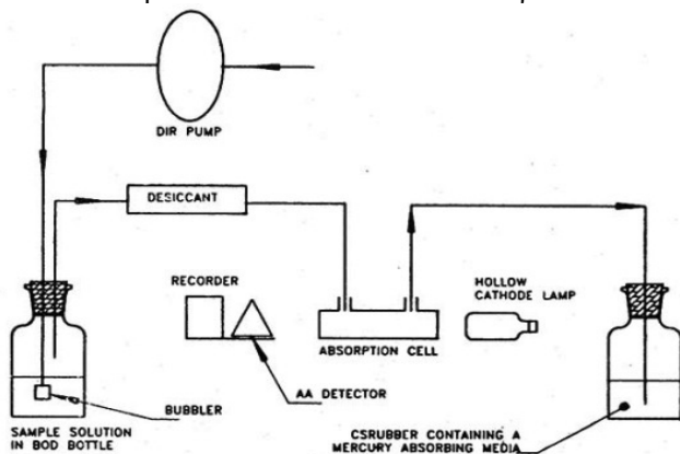
Figura 1. Diagramë skematike e sistemit CVAAS për avullimin dhe atomizimin e mërkurit
